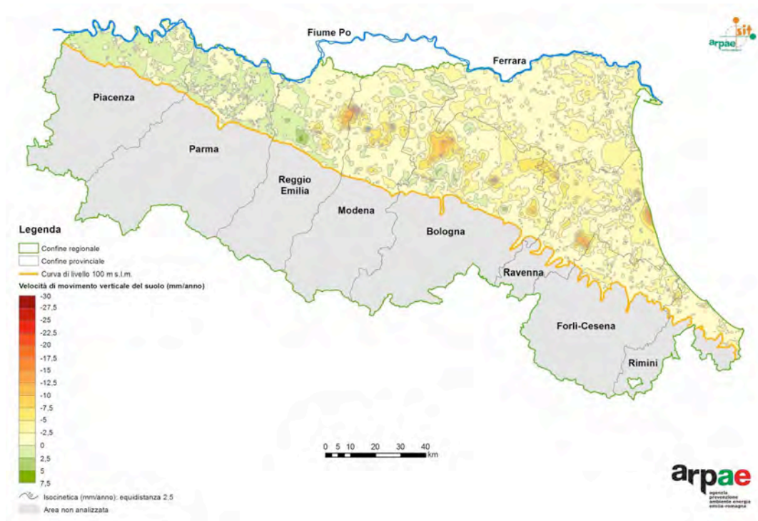
Figura 61 - Velocità di movimento verticale del suolo nel periodo 2011-2016 (ARPAE Emilia-Romagna)
